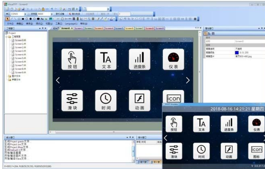
图 10-1 VisualTFT 主界面
