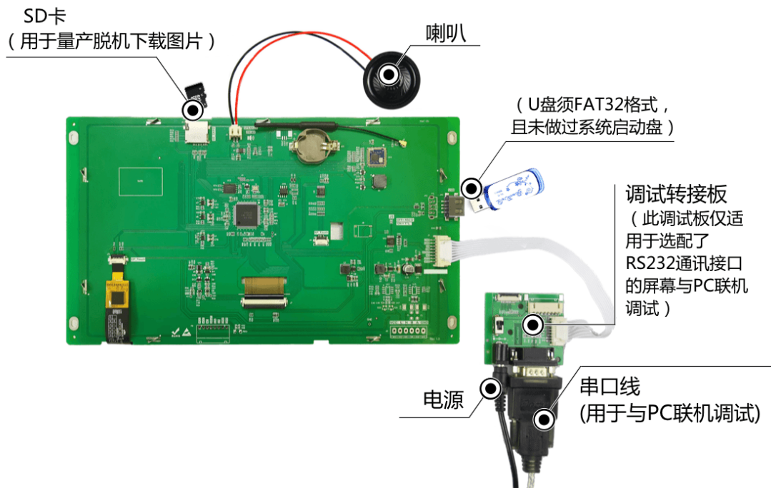
图 1-6 调试工具
