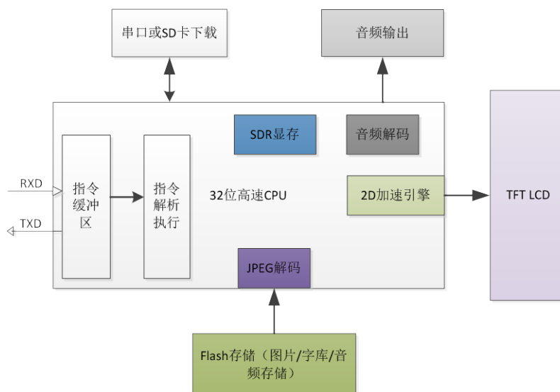
图 9-1 物联型串口屏内部结构图
