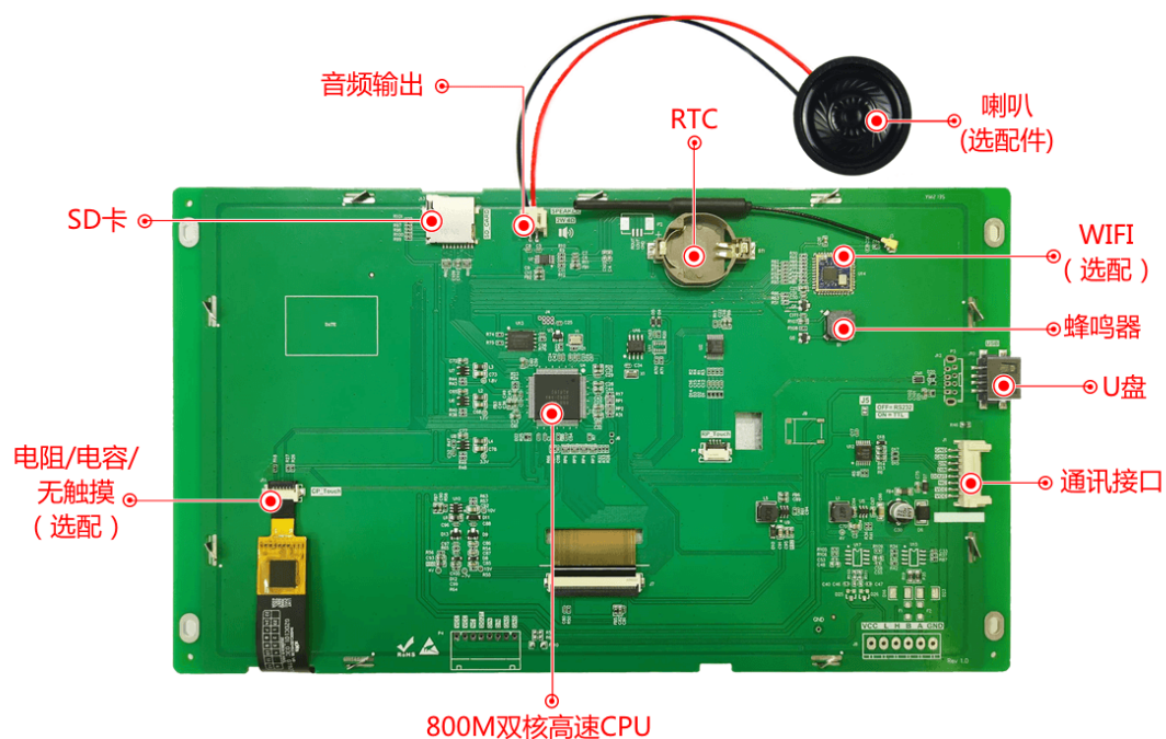
图 1-4 硬件配置图
