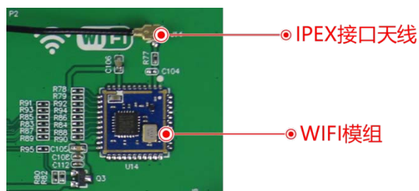
图 1-5 WIFI 配置图
